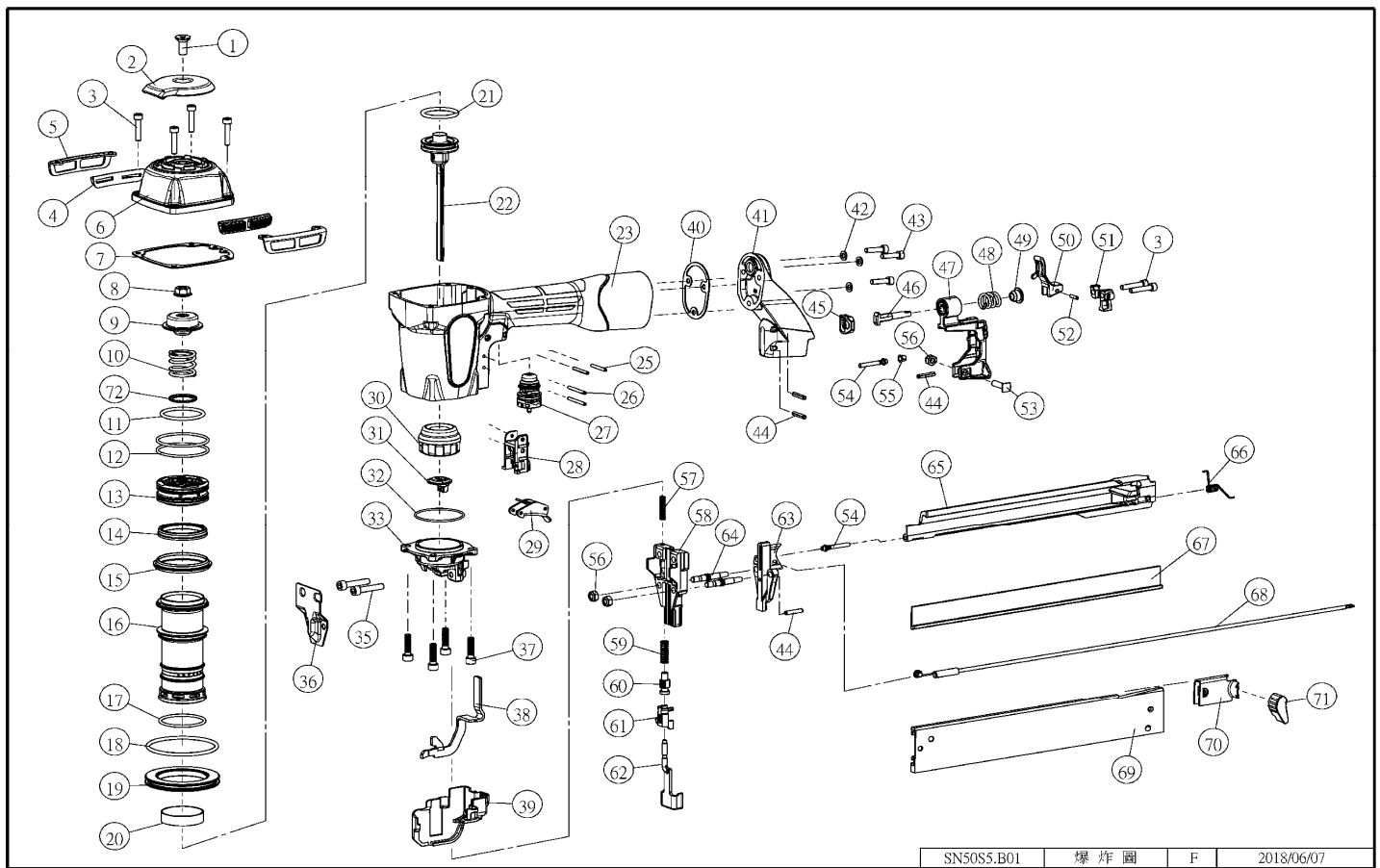
SN50S5.B01 爆炸圖 F 2018/06/07
