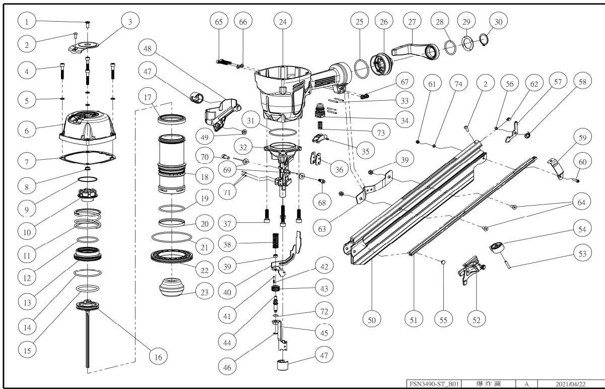
FSN3490-ST_B01 爆炸圖 A 2021/04/22
